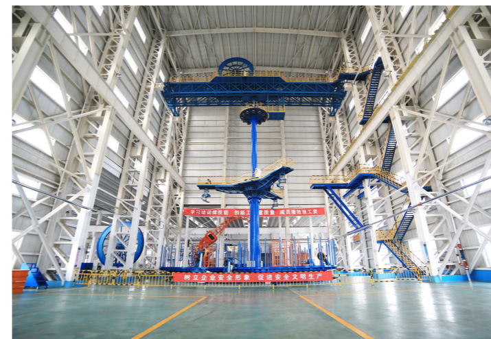
海缆公司可连续不间断开车,保证了大长度海底电缆的生产;拥有10000mm/3+3150/12型超大型立式成缆装设备,可连续生产≥45公里无接头。
